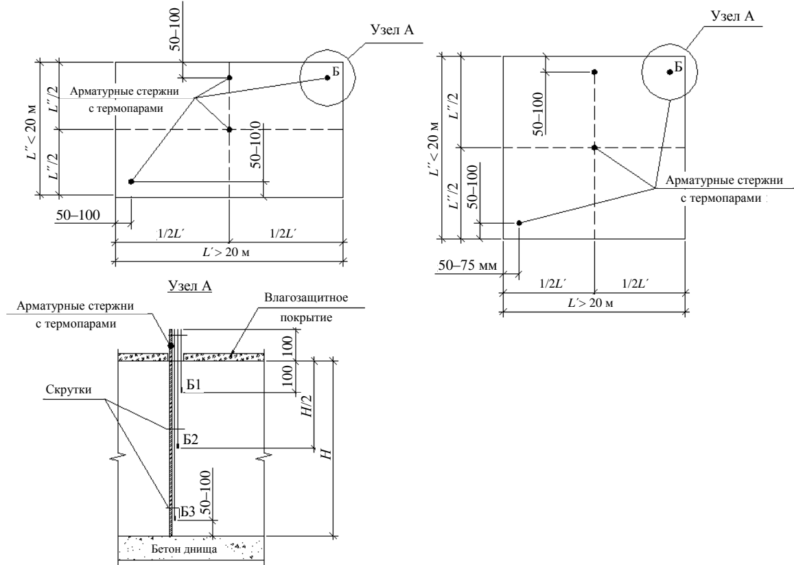
План фундаментной плиты (вид сверху)
