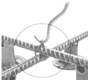
Рисунок 7.3 – Вязка арматуры крючком
